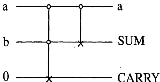
Fig. 6.4 An Adder
