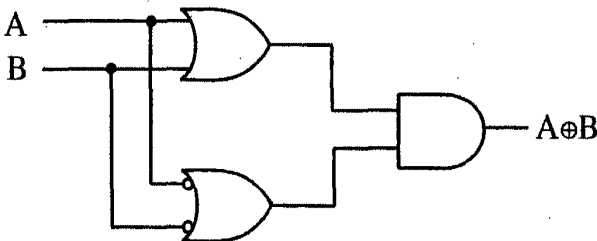
Fig. 2.10 An Alternative XOR
