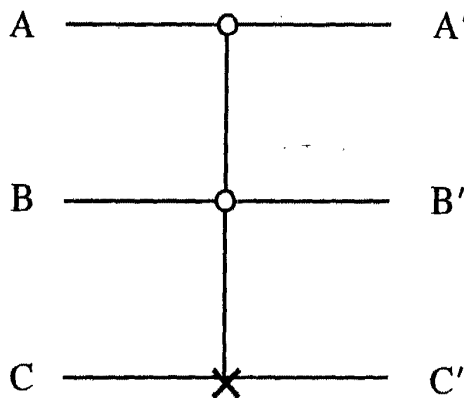
Fig. 2.22 The CCN Gate
