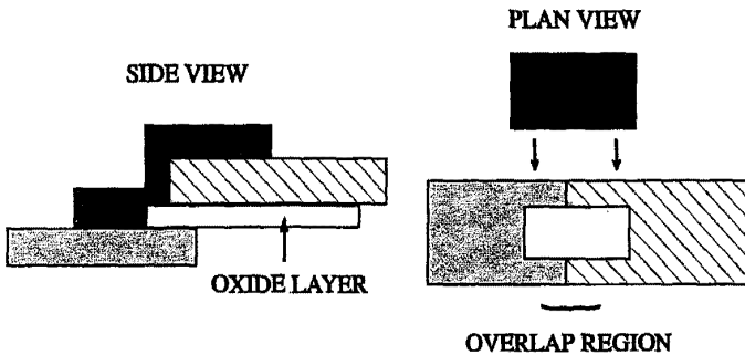
Fig. 7.52 Polysilicon-Diffusion Layer Contact
