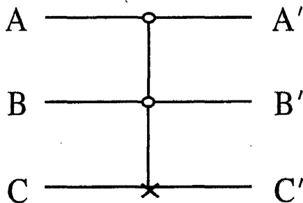
Fig. 5.10 The CCN Gate
