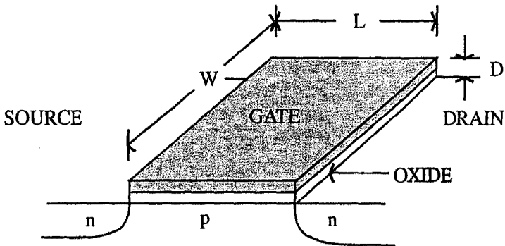
Fig. 7.8 The MOSFET
