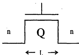
Fig. 7.44 The Simple MOSFET
