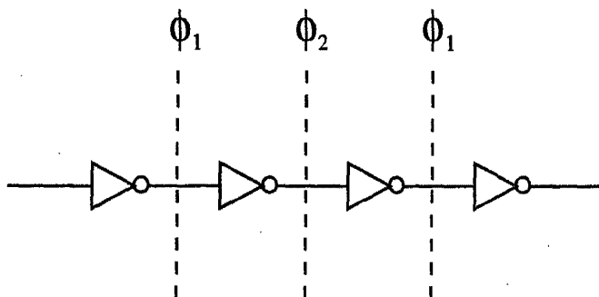
Fig. 7.60 A Shift Register
